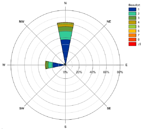
Κατεύθυνση και συχνότητα έντασης ανέμων Μέσες τιμές των καλοκαιρινών μηνών ετών 1960-2004 (Σταθμός Παλαιόχωρας)
